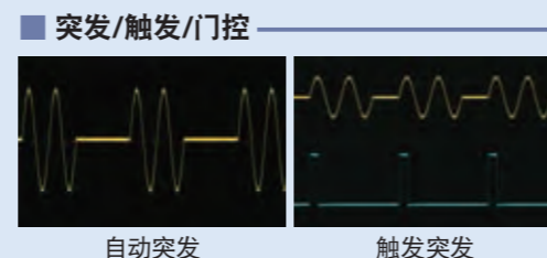
自动突发 触发突发
