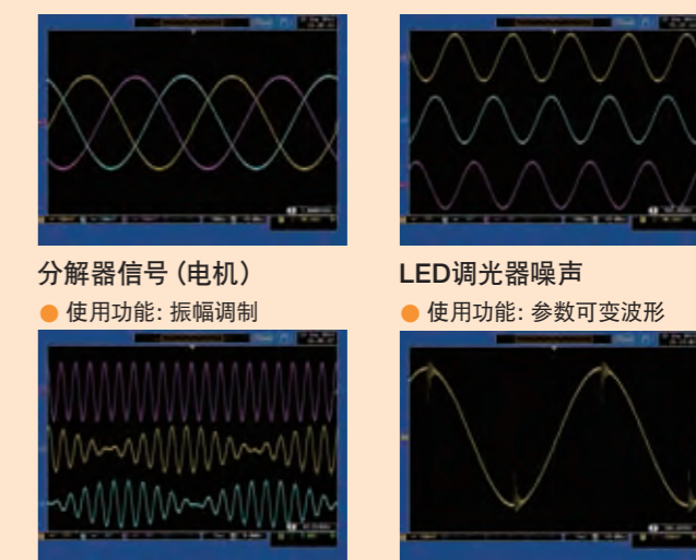
振幅调制正弦波后从CH1输出，CH2输出调制相位前进90°的信号。
