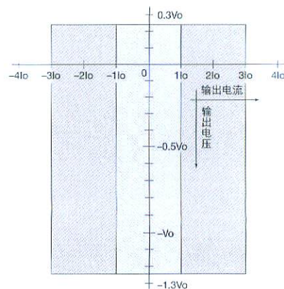
适用于HSA4012, HSA4014的+25V、-125V范围 以及HSA4051, HSA4052的+50V、-250V范围
