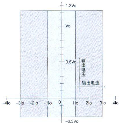
适用于HSA4012, HSA4014的+125V、-25V范围 以及HSA4051, HSA4052的+250V、-50V范围
