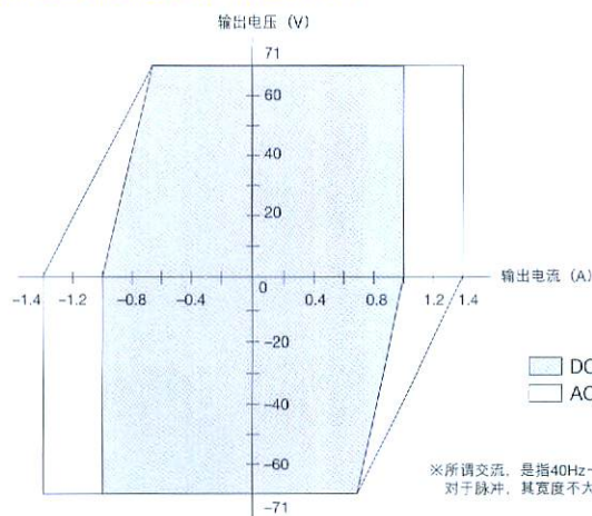
适用于HSA4012, HSA4014的±75V范围 HSA4051, HSA4052的±150V范围 以及HSA4011 (虚线部分)
