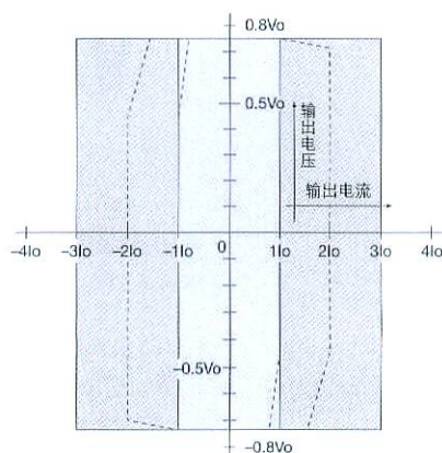
适用于HSA4012, HSA4014的±75V范围 HSA4051, HSA4052的±150V范围 以及HSA4011 (虚线部分)
